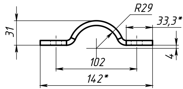
Поз.4 (Полухомут)
